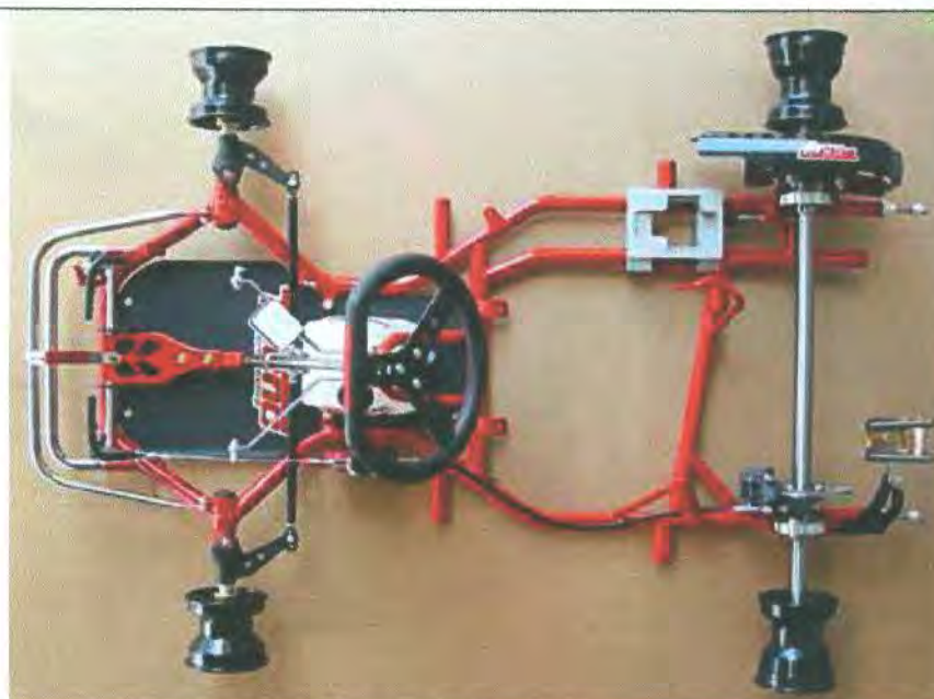
Вид сверху шасси в комплекте с рулевым управлением, педалями, топливным баком, полом, задней осью, колесными дисками, креплением двигателя (опционно), но без сиденья, шин, бамперов и кузова (пластика) Insert plan view of chassis with complete steering, pedals, fuel tank, floor, rear axle, rims, engine support; but without seat, tyres, bumpers or bodywork
