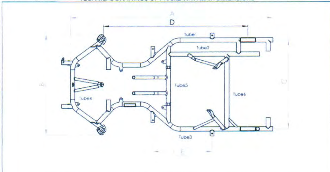
Вид сверху в масштабе 1:10 с размерами таблицы 1 (рама со всеми стяжками и подставками) Top view in scale 1:10 with labels of table 1 (frame with all brackets and supports)
