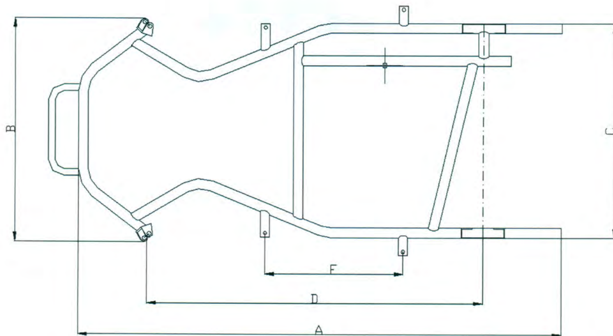
Вид сверху в масштабе 1:10 с размерами таблицы 1 (рама со всеми стяжками и подставками) Top view in scale 1:10 with labels of table 1 (frame with all brackets and supports)
