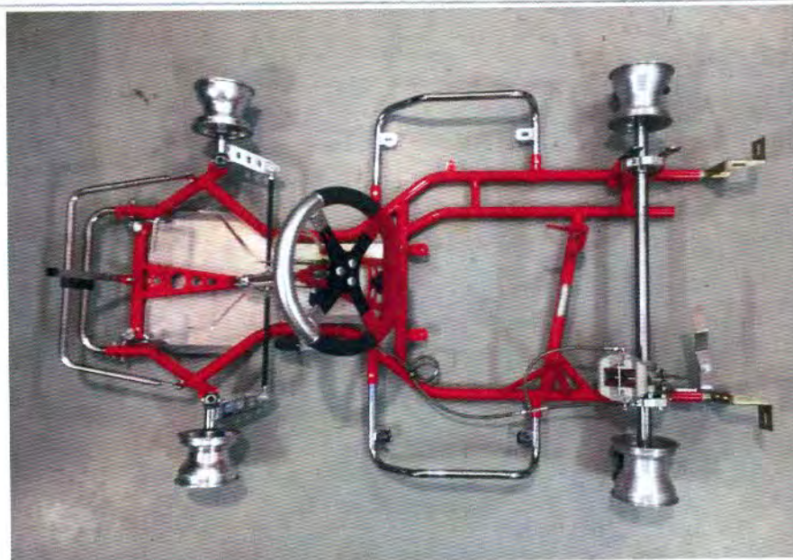
Фотография шасси без сиденья, шин, бамперов и кузова (Photograph of the chassis less seat, bumpers and bodywork)
